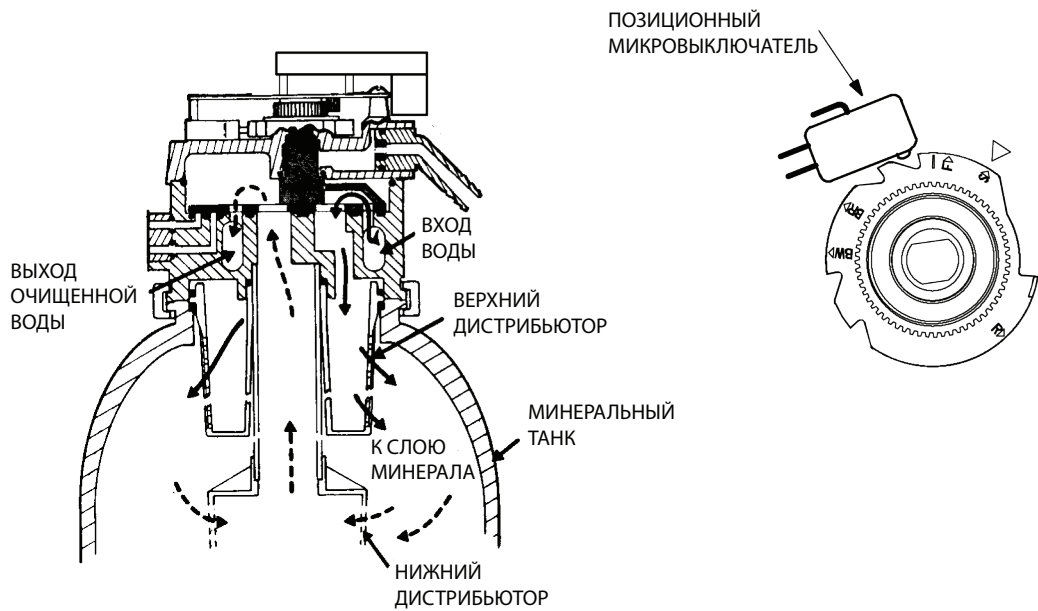
Рис. 10. Сервисный цикл
