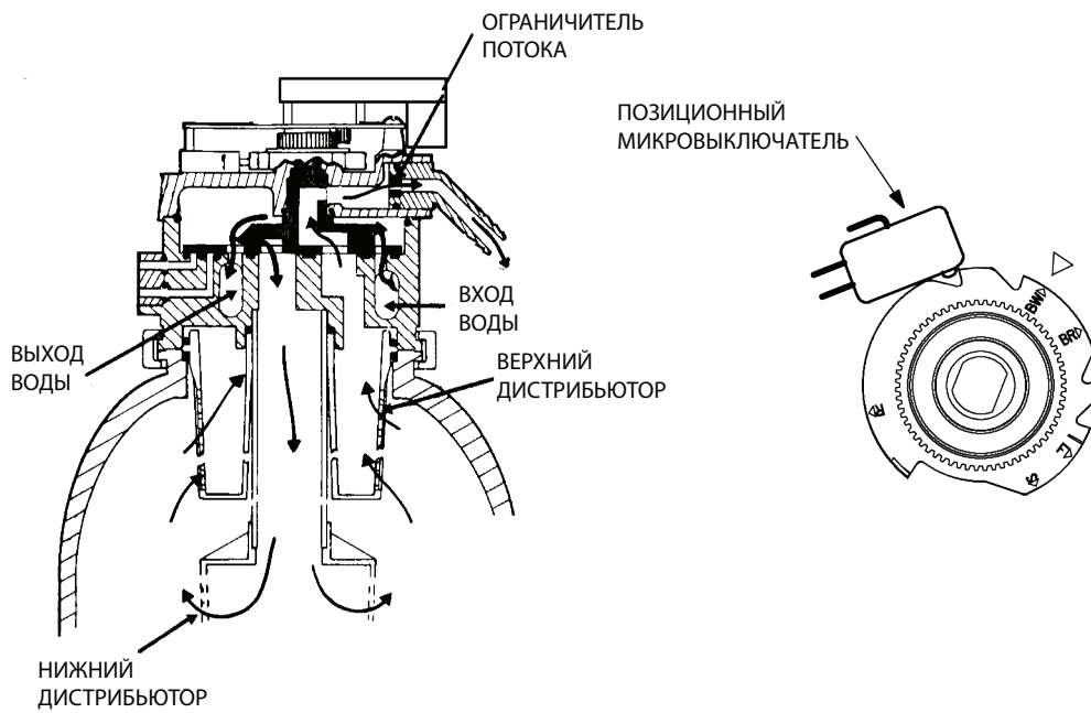
Рис. 11. Обратная промывка
