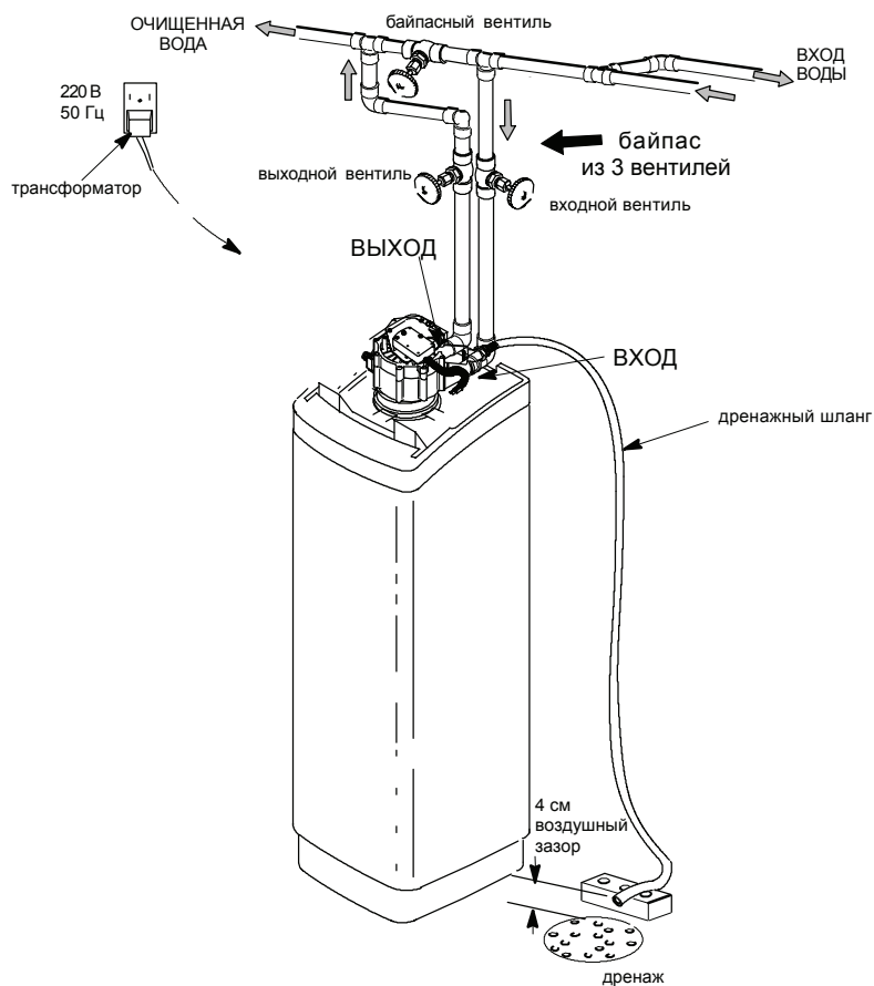
Рис. 2. Типовая схема установки
