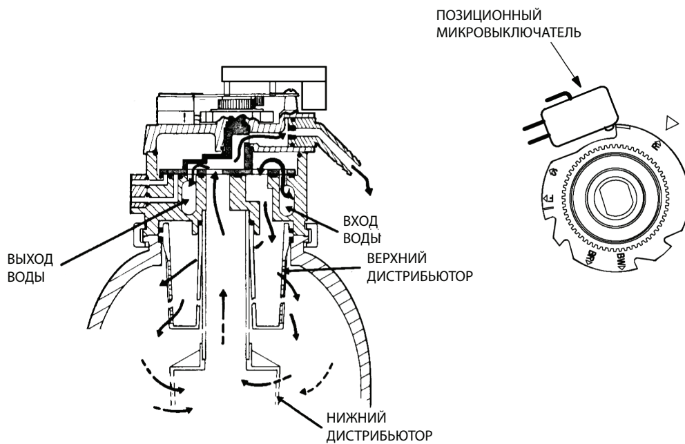
Рис. 12. Быстрая промывка
