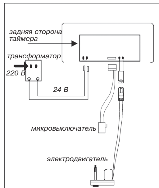
Рис. 8. Электронный таймер
