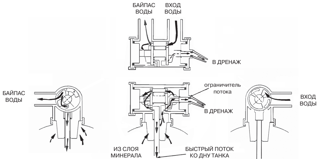
Рис. 11. Обратная промывка
